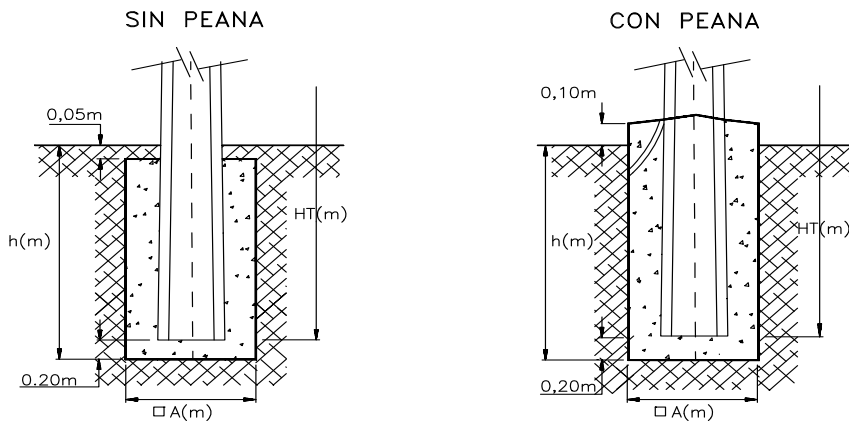
DETALLES DE CIMENTACION (Figura 7)
