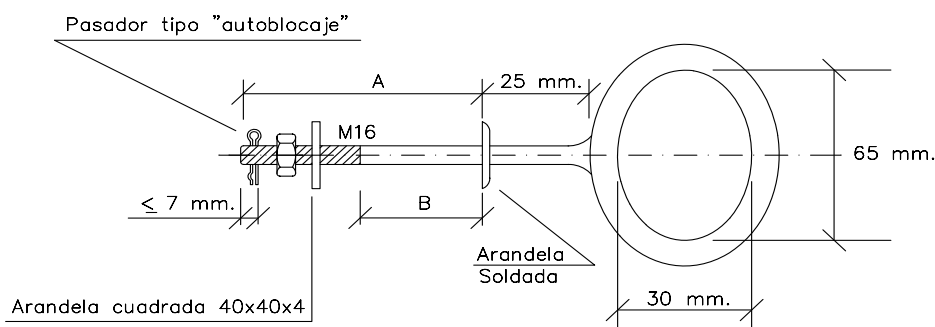
TORNILLO PASANTE DE ANILLA OVALADA PARA LINEA DE VIDA (Figura 3)
