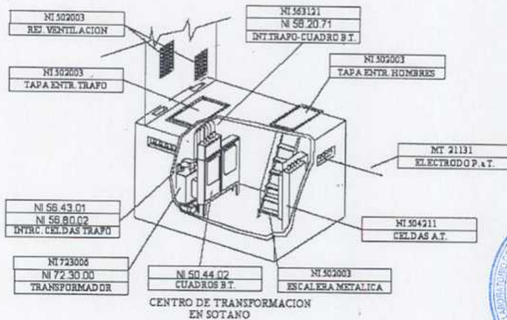
Figura 4 Tipo Sótano
