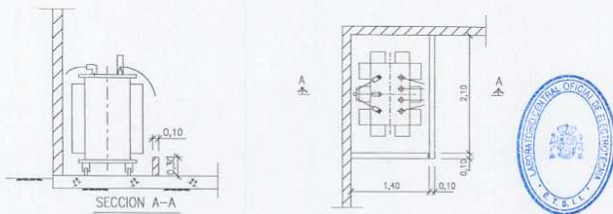
Figura 1. Foso bañera
