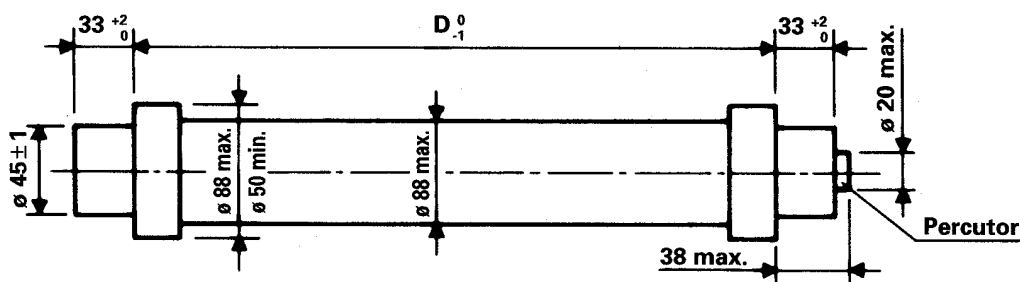
Fig. 1: fusible limitador
