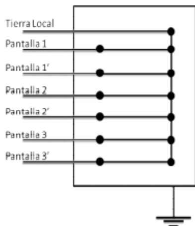
Esquema 3: Caja de puesta a tierra directa de todas las pantallas.
