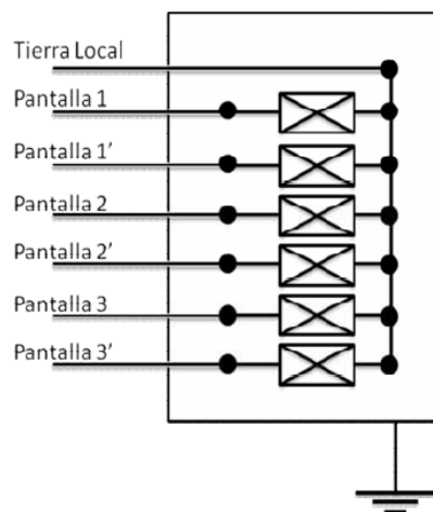
Esquema 4: Caja de puesta a tierra de todas las pantallas a través de limitadores de tensión.
